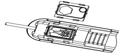
Figura 3 Una vez insertado el cable de alimentación, realice la conexión L(Linea) N(Neutro) a la regleta de la luminaria, luego coloque la tapa a presión.
